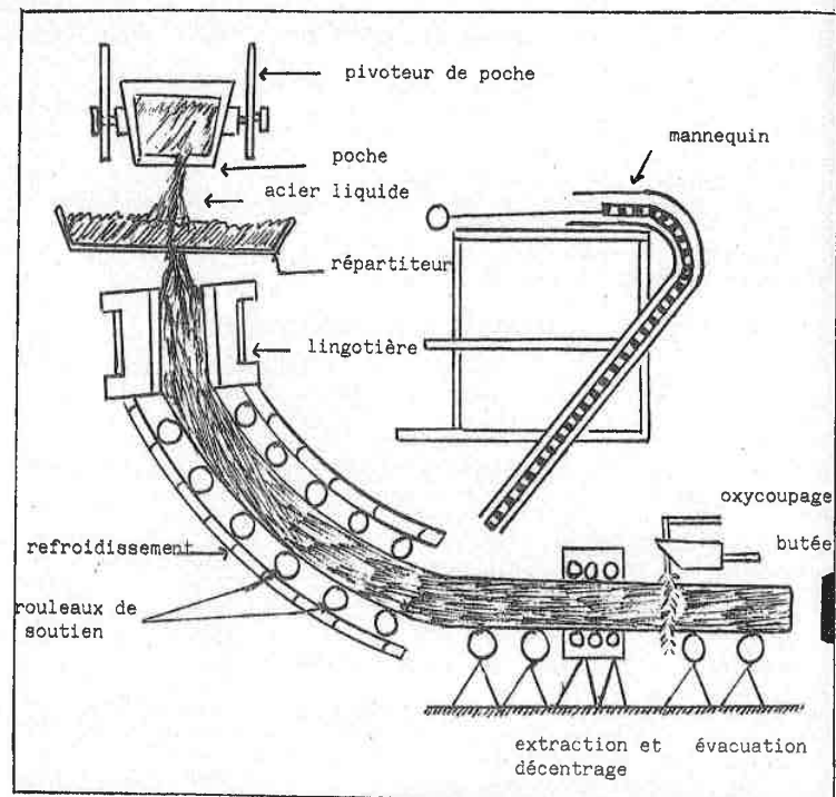
Structure générale d'une ligne de coulée continue
