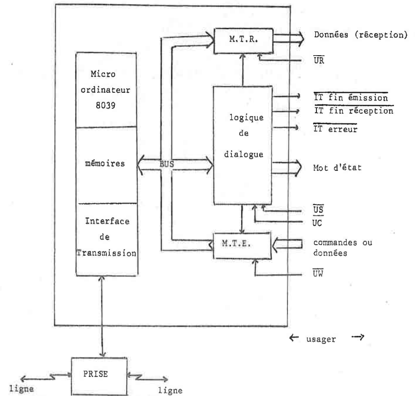
Synoptique du TR 81 A
