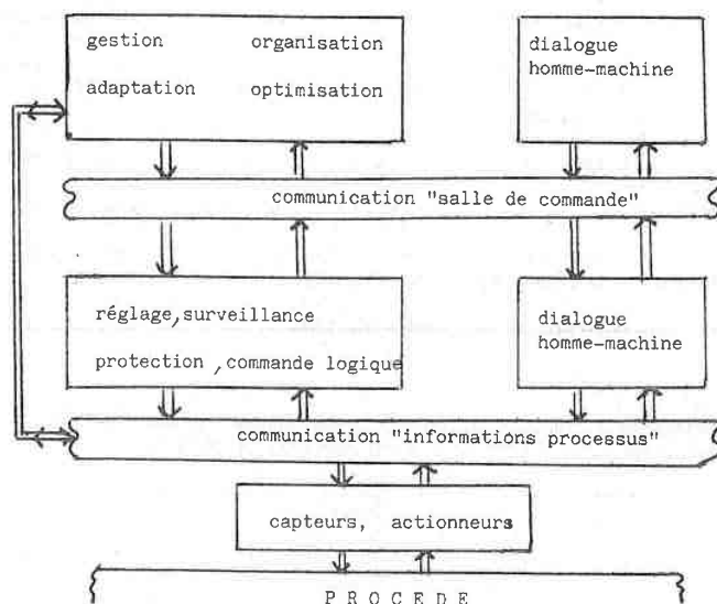
Hiérarchisation des communications dans une ACPI
