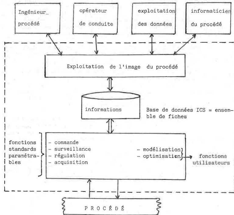
Architecture d'un système utilisant ICS
