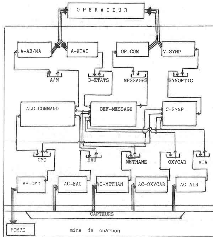
Application de commande de la pompe et son environnement
