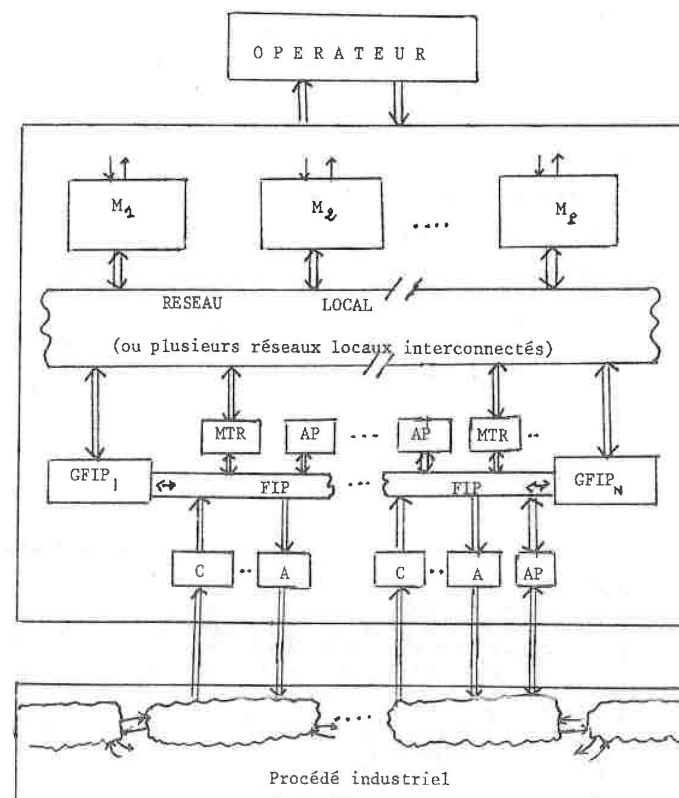
Architecture d'une installation de commande utilisant FIP
