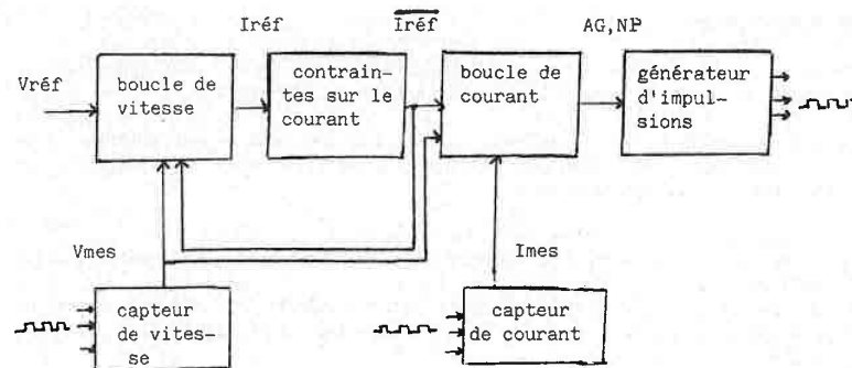
structure de régulation du moteur
