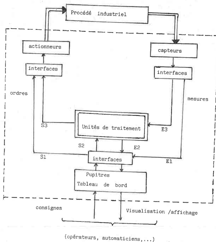
(opérateurs, automaticiens,...) Architecture d'un système de commande de PI
