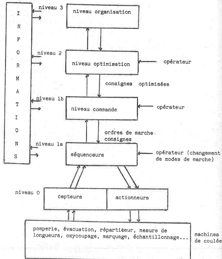
Structure hiérarchisée de la commande de la coulée continue
