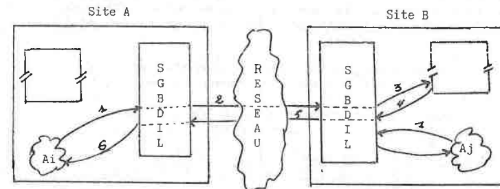
Circuit d'accès à une donnée
