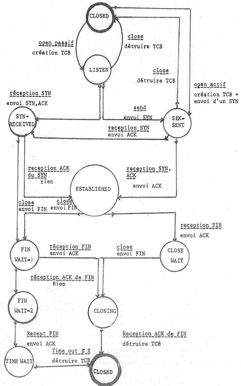
Diagramme des états d'une connexion
