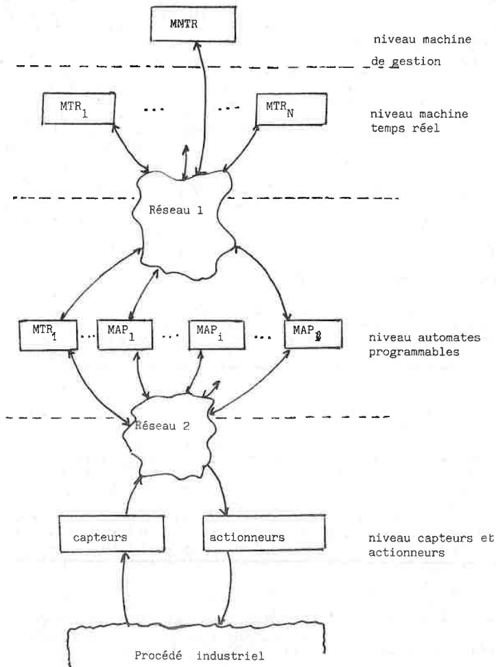
Hierarchisation des équipements dans une ACPI complexe
