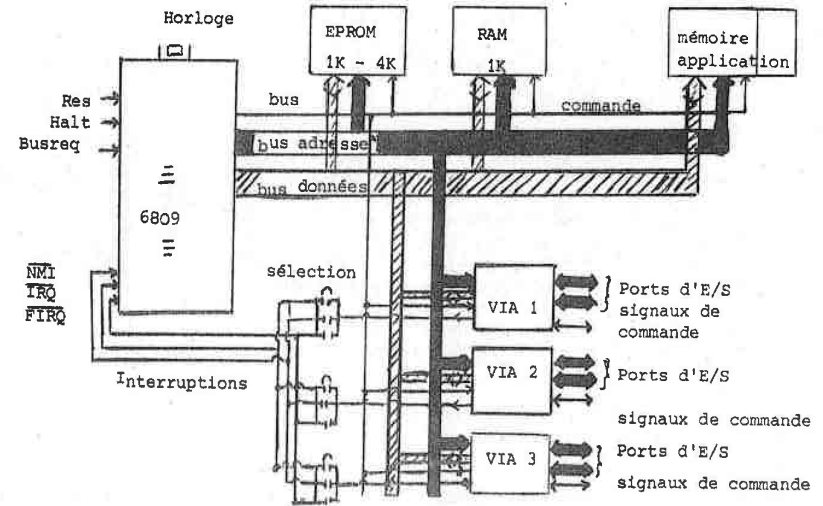
SYNOPTIQUE DU MODULE MPU9
