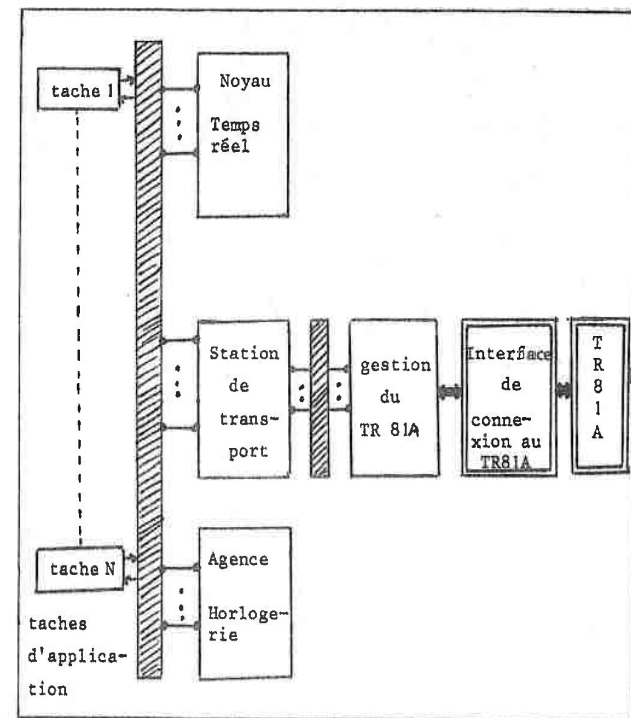
Structure d'une station
