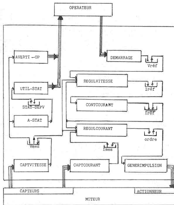
Schéma de l'application et de son environnement
