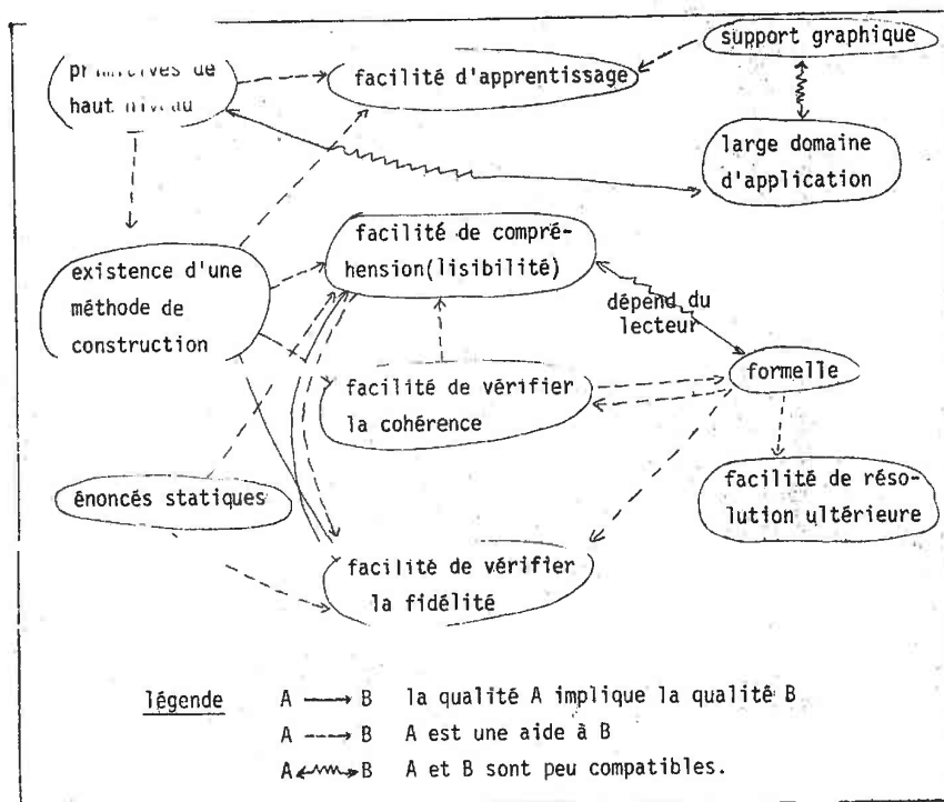
figure 13 - lien entre les différentes qualités d'un langage de spécification
