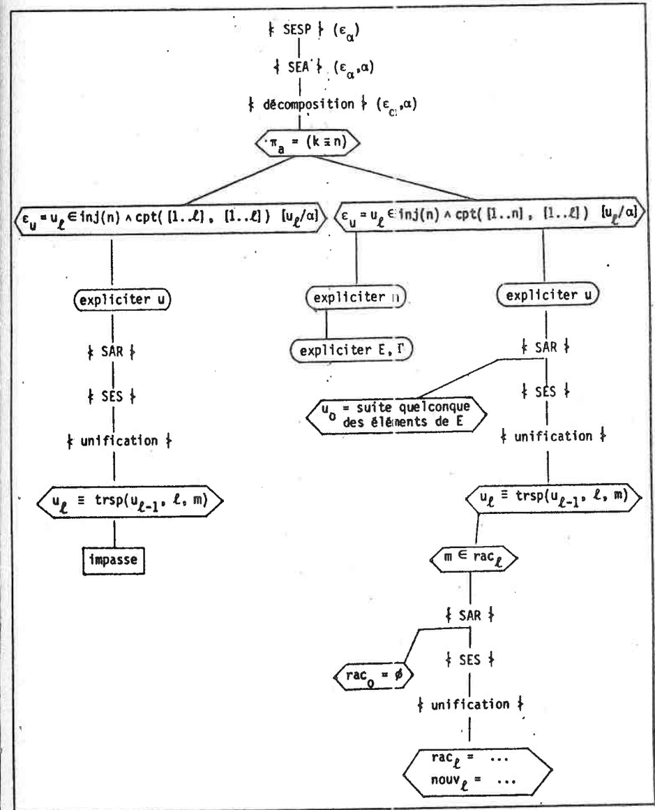
Figure 3 : Arbres de choix du tri topologique
