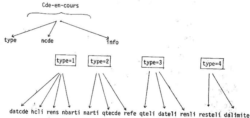
Figure 4 : enregistrements de cde-en-cours
