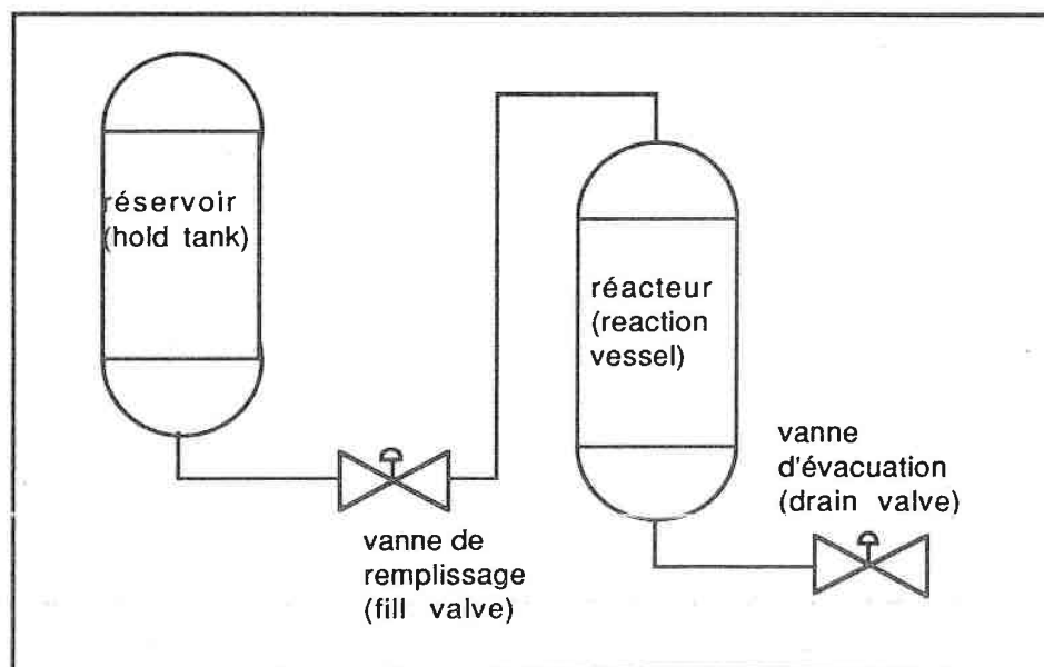
exemple du système de contrôle d'un réacteur [War 88]
