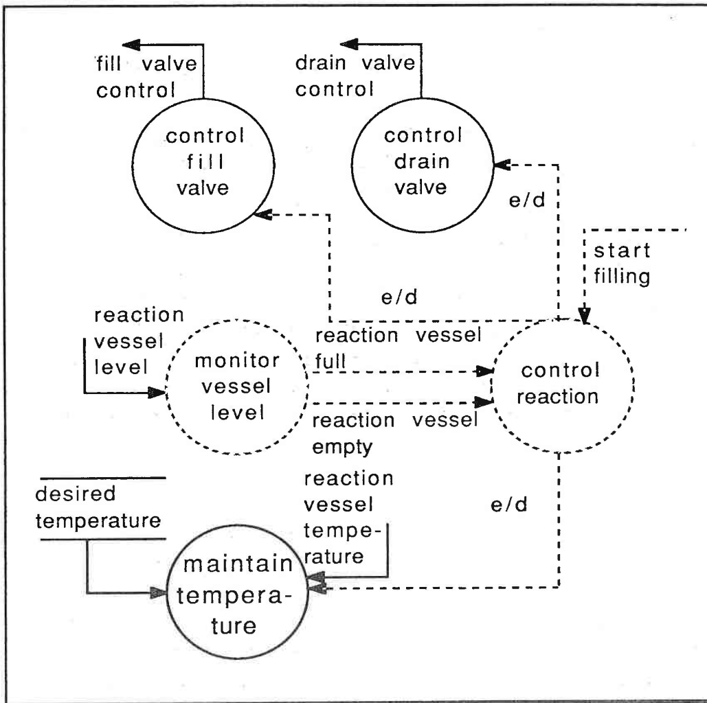
spécification fonctionnelle proposée par Ward selon le formalisme Ward-Mellor [War 88]
