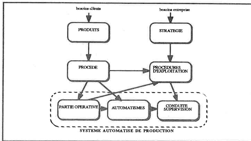
les éléments déterminants dans la définition de l'Architecture d'un SAP.
