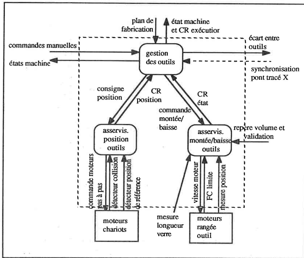
schéma de structure fonctionnelle de la conduite automatique du pont de tracé longitudinal (DECPTY)
