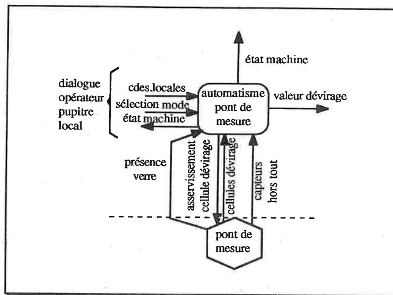
structure fonctionnelle de la fonction de suivi de dévirage (MESDEV)
