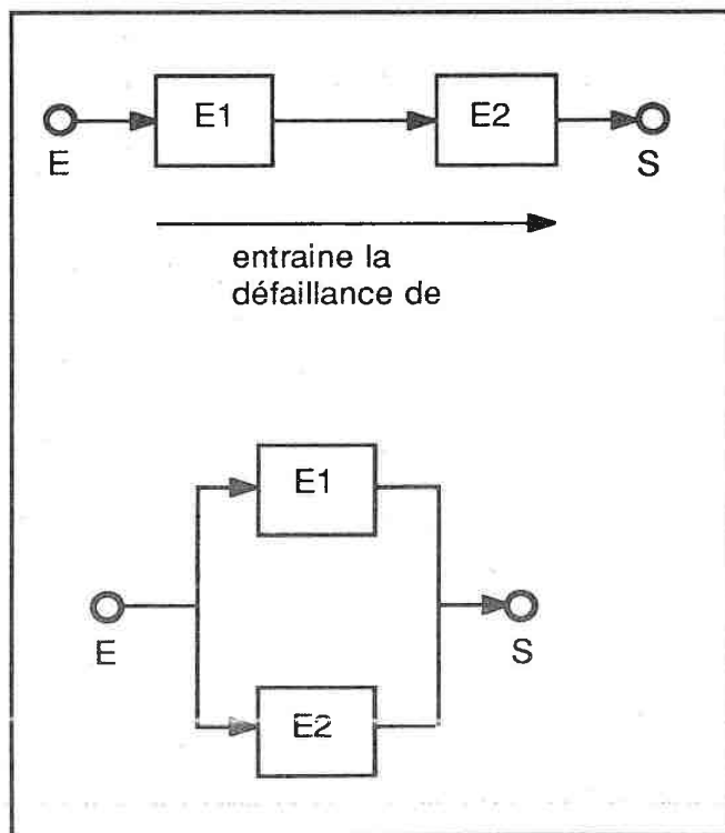
les diagramme série et parallèle de fiabilité
