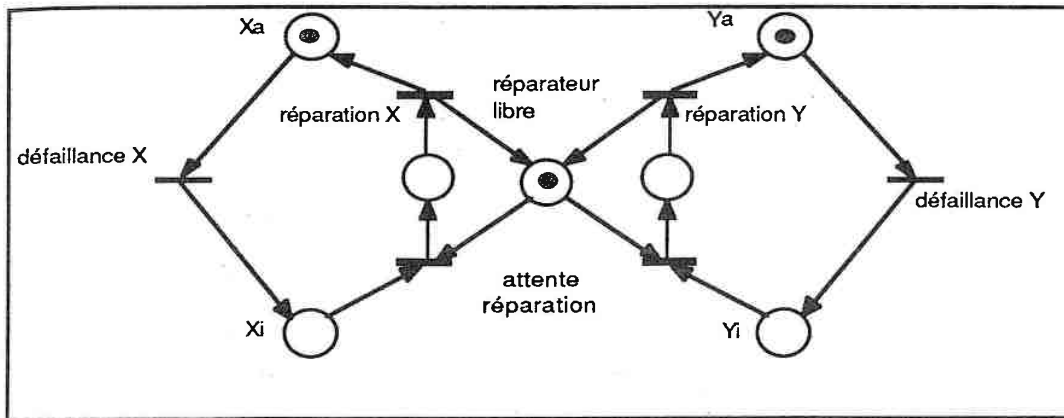
le réseau de Petri stochastique d'un système à deux composants avec un seul réparateur partagé FIFO
