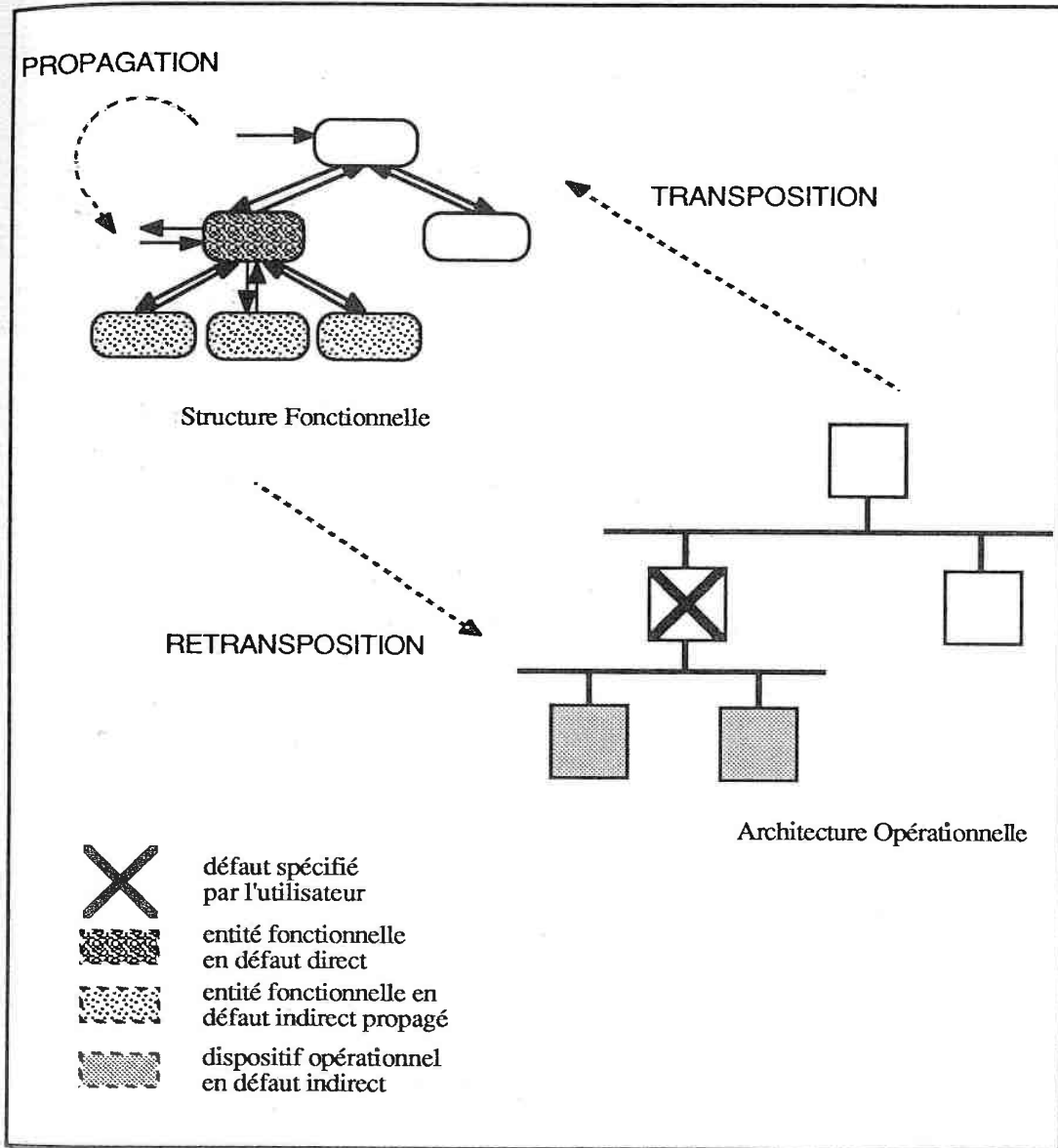
les trois phases de la procédure d'analyse des effets de défaillances
