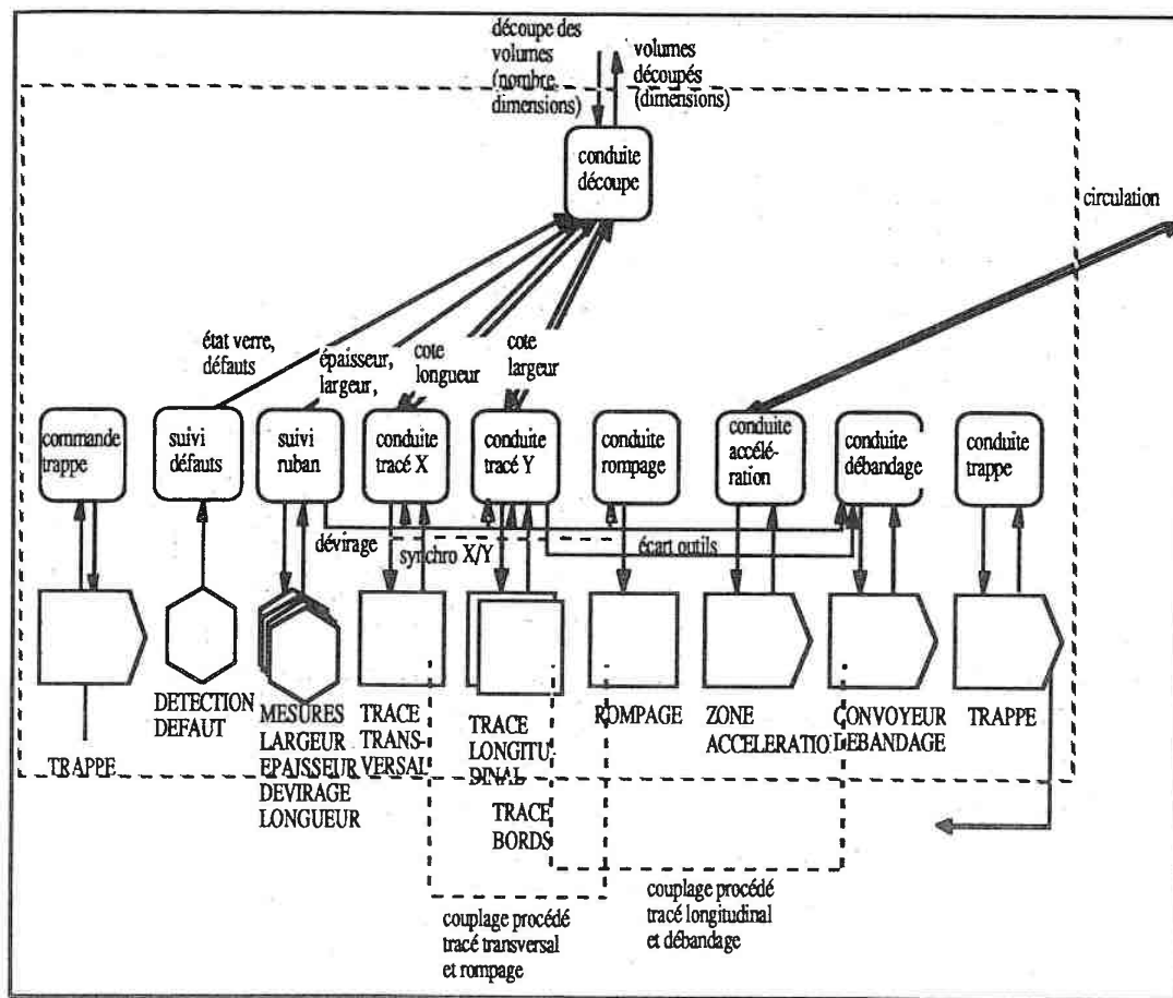
schéma de la structure fonctionnelle (niveau 2) de la conduite automatique du centre de découpe
