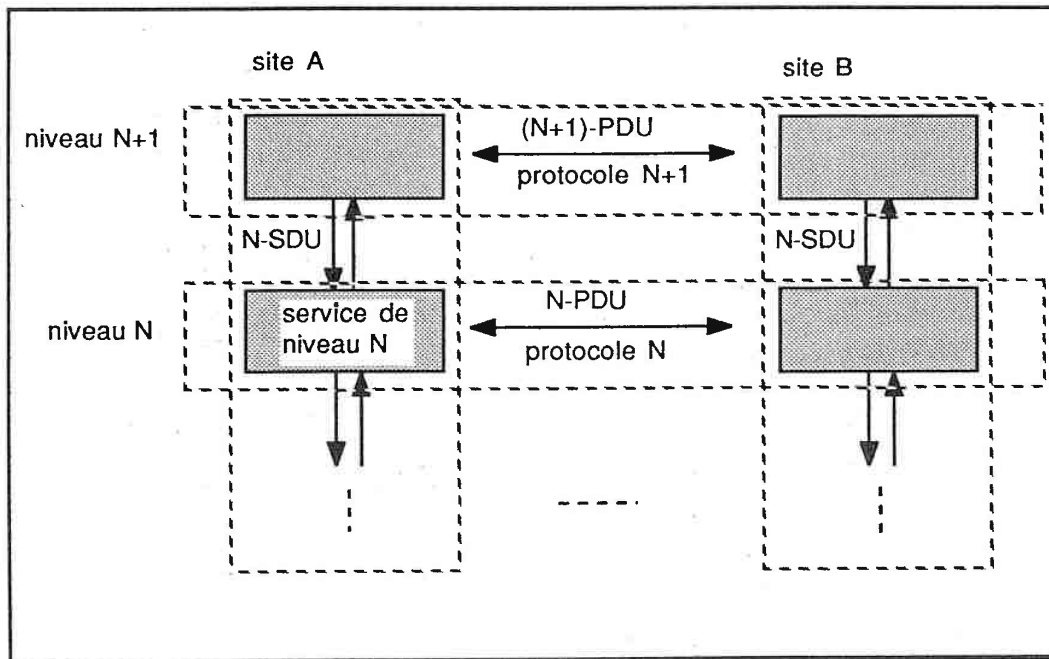
services et protocoles de communication dans le modèle OSI de l'ISO
