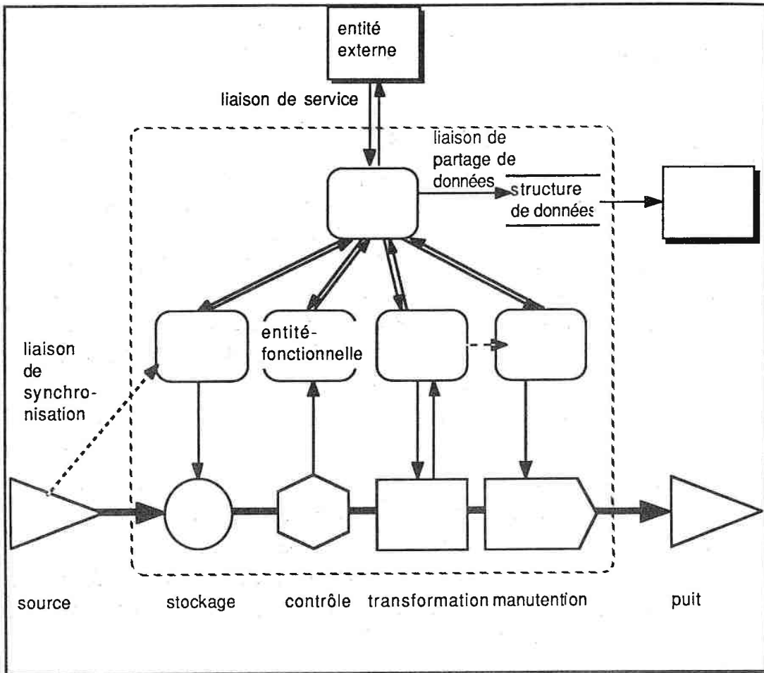
les éléments du modèle générique de structuration fonctionnelle du SAP
