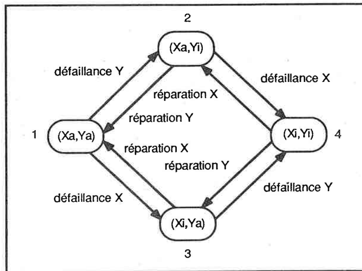
le graphe de Markov d'un système réparable à deux composants ayant chacun un réparateur
