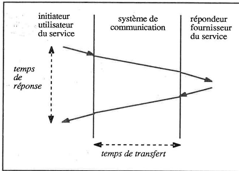
temps de réponse au niveau application et temps de transferts réseau
