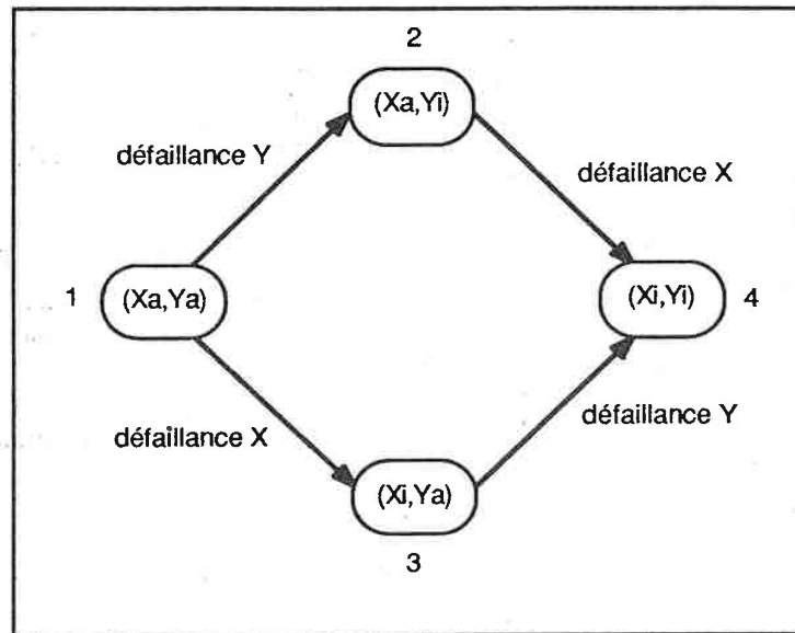
le graphe de Markov d'un système non-réparable à deux composants
