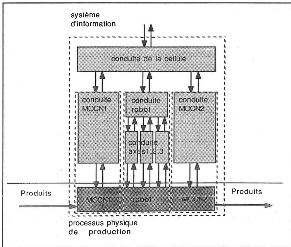
exemple de modélisation avec le concept de service d'une cellule de fabrication
