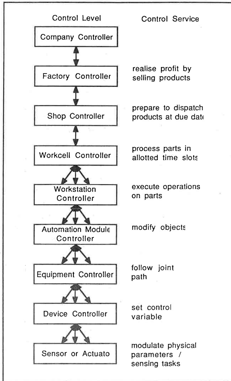
les 8 niveaux du modèle CAM-Centre Philips proposé par Biemans
