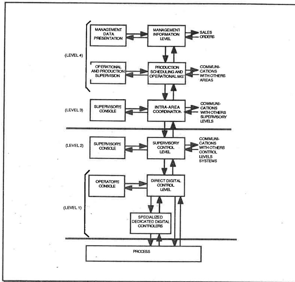
les 4 niveaux proposés dans le modèle de l'université de Purdue
