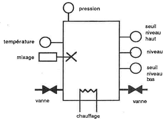
les équipements d'un réservoir
