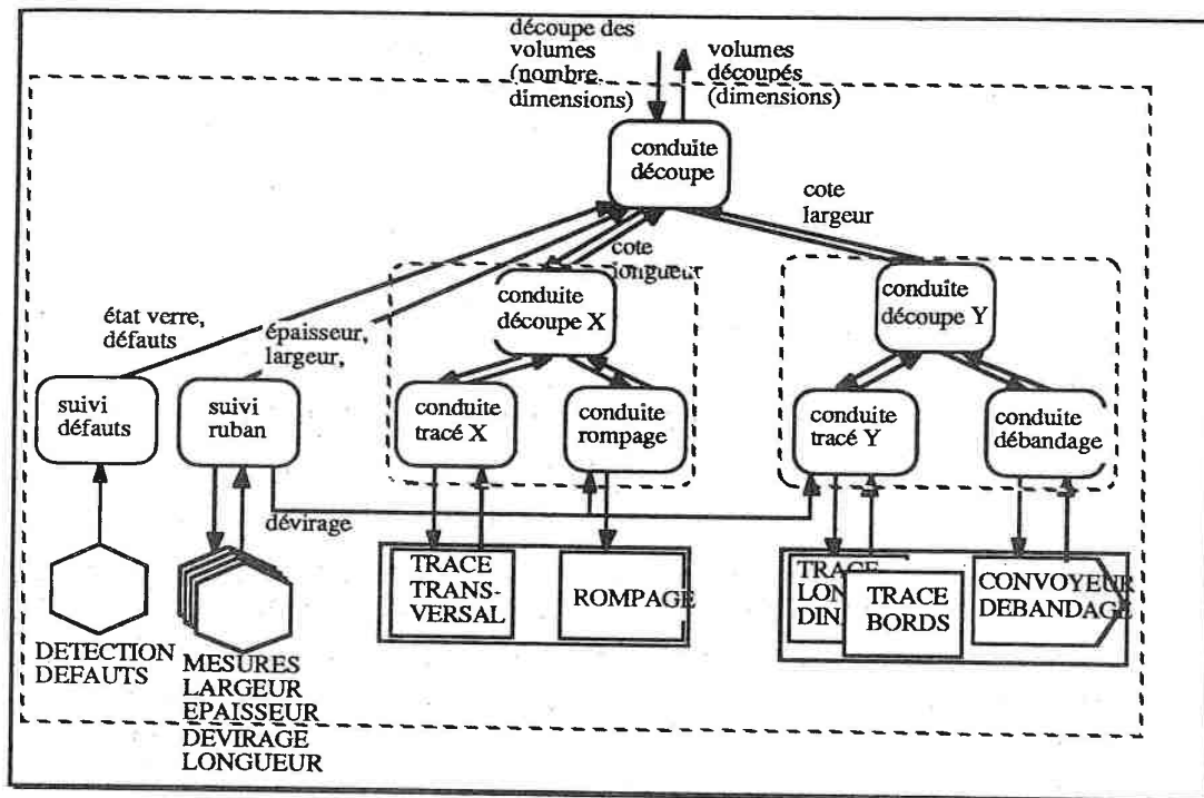
schéma (simplifié) de la structure fonctionnelle (niveau 1) de la conduite automatique du centre de découpe
