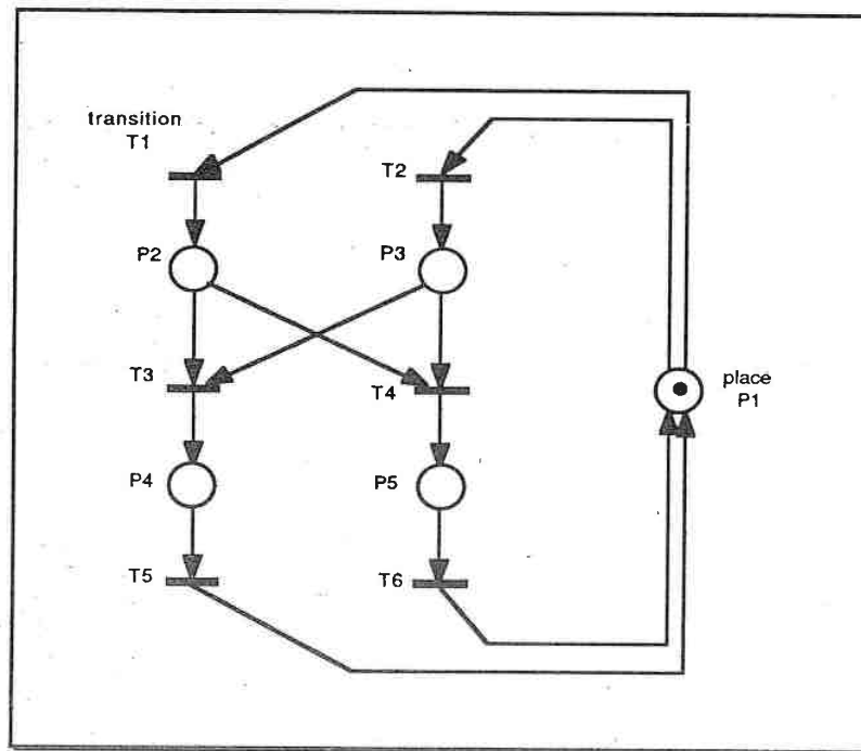
exemple de Réseau de Petri
