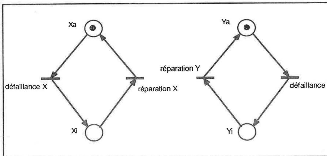
le réseau de Petri stochastique d'un système à deux composants avec chacun un réparateur
