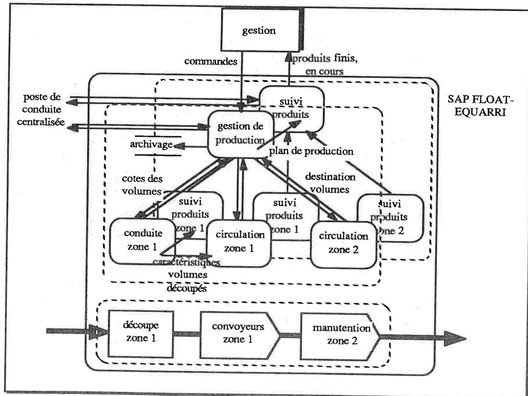
schéma de structure fonctionnelle de niveau 1 du SAP FLOAT (schéma de contexte)
