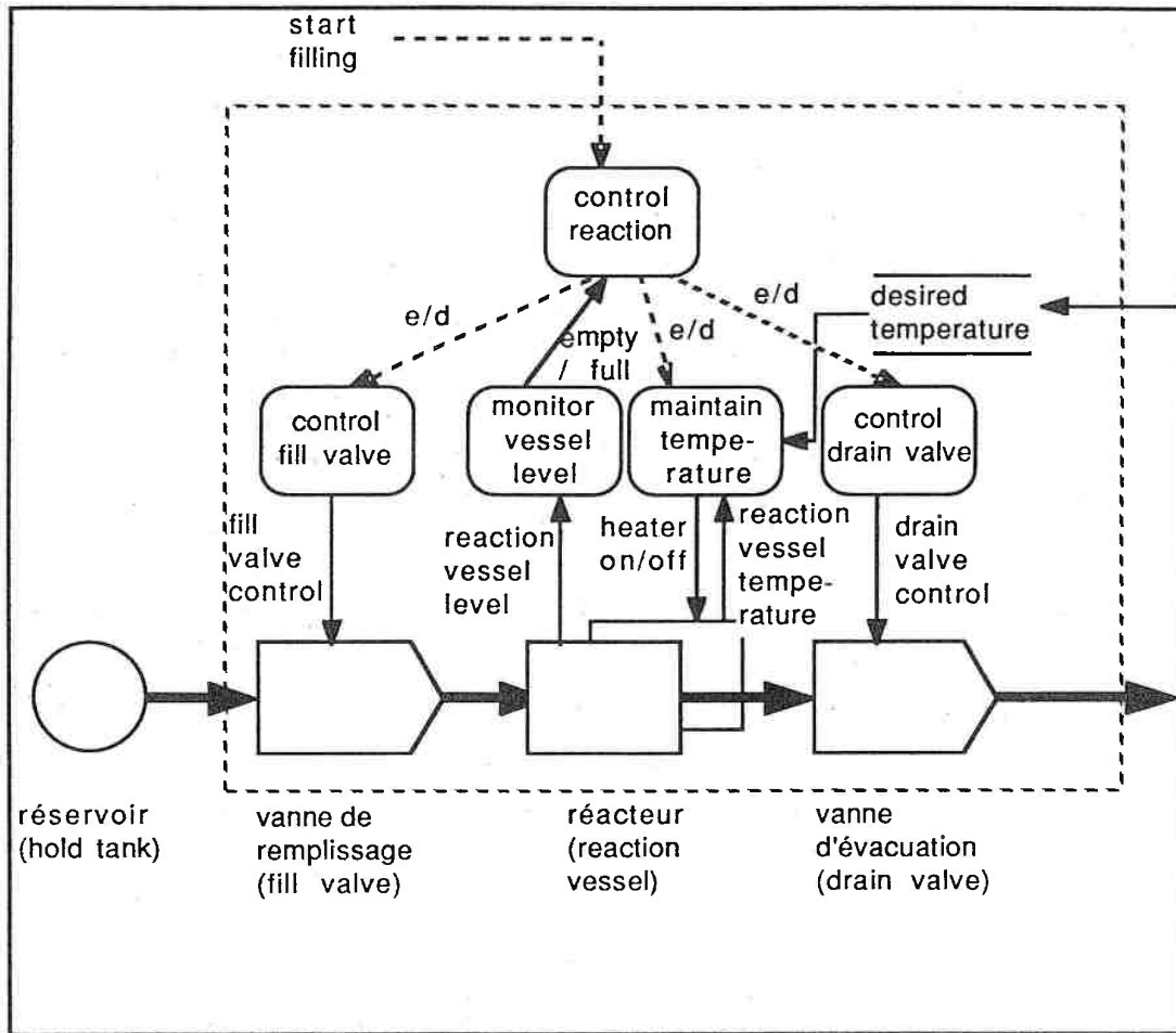
Structuration Fonctionnelle de 2 ème niveau de l'exemple du système de contrôle d'un réacteur
