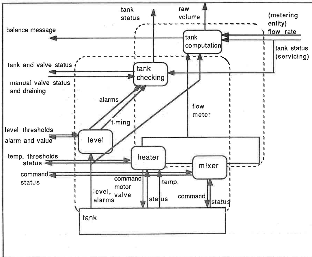
schéma fonctionnel de l'entité reservoir
