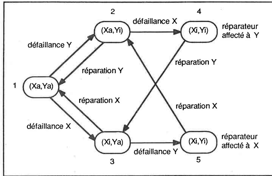
le graphe de Markov d'un système réparable à deux composants avec un seul réparateur géré en FIFO
