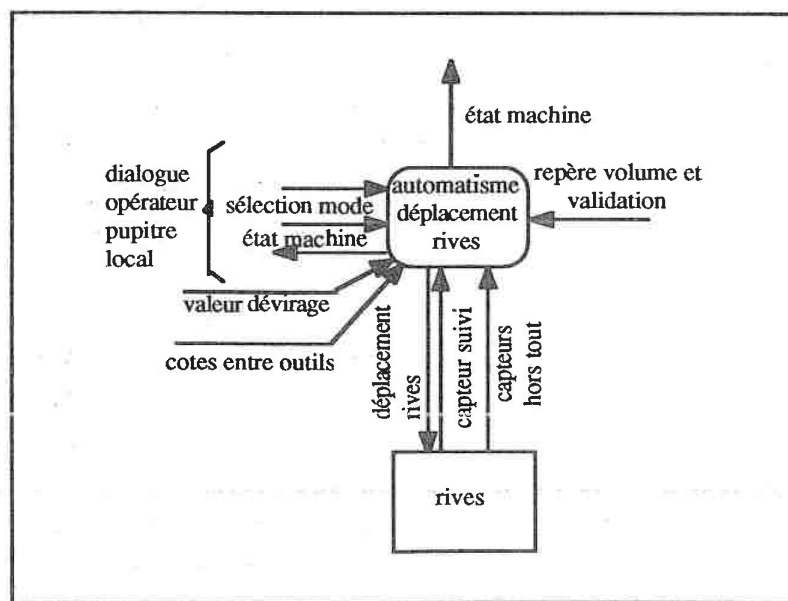
schéma de structure fonctionnelle de la conduite du déplacement des rives de débandage (MILARI)
