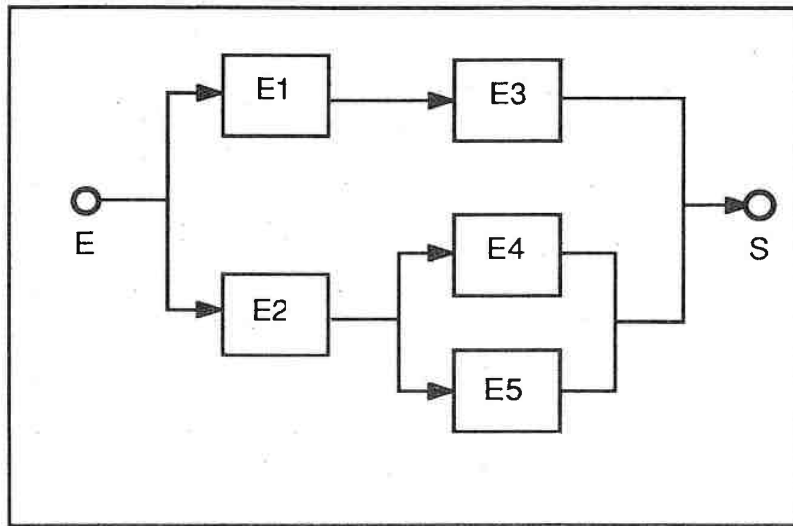
un exemple de diagramme de fiabilité
