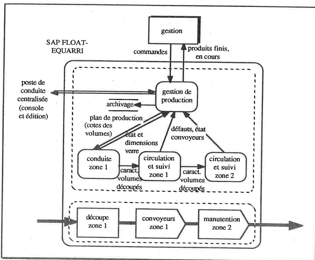
schéma de structure fonctionnelle de niveau 2 du SAP FLOAT (schéma de contexte)
