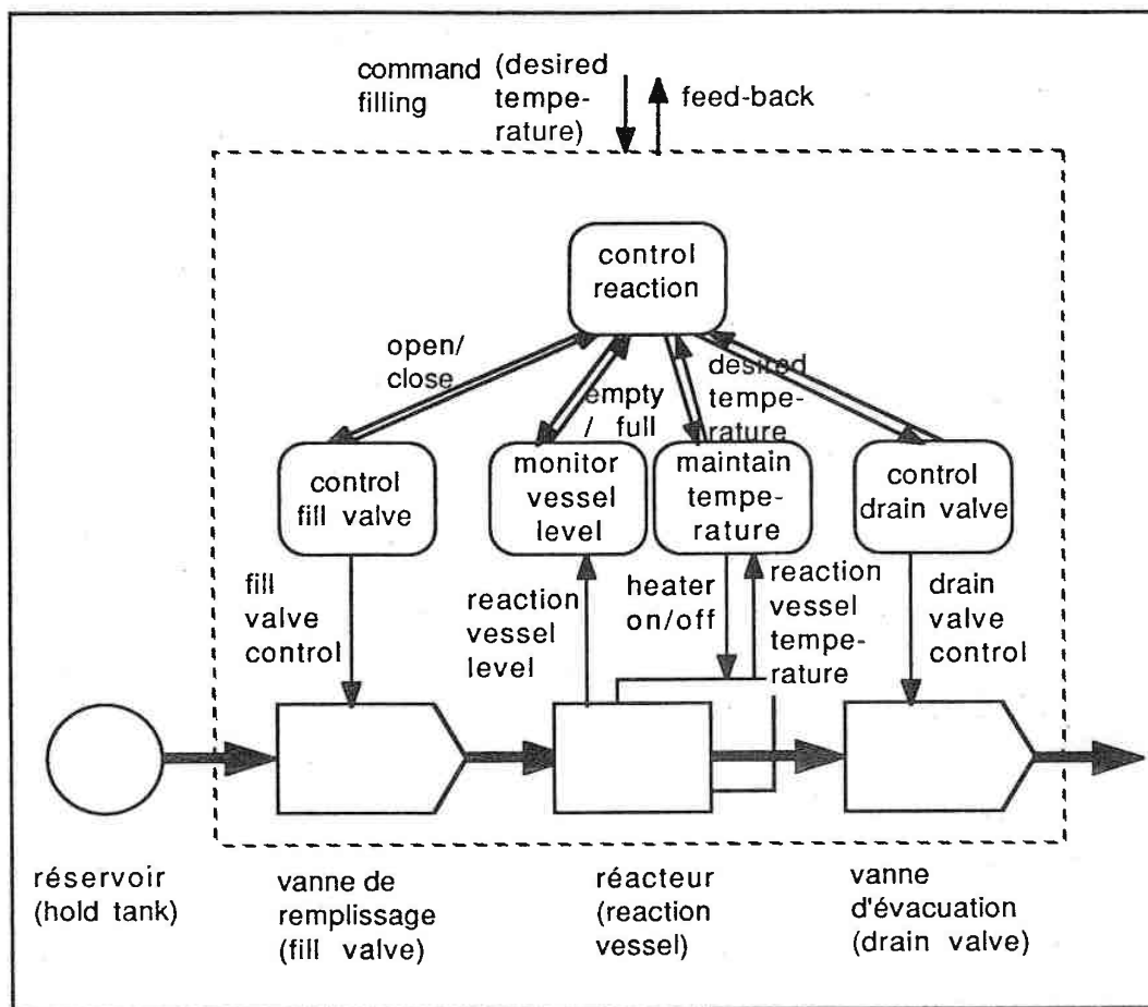
Structuration Fonctionnelle de 1 er niveau de l'exemple du système de contrôle d'un réacteur
