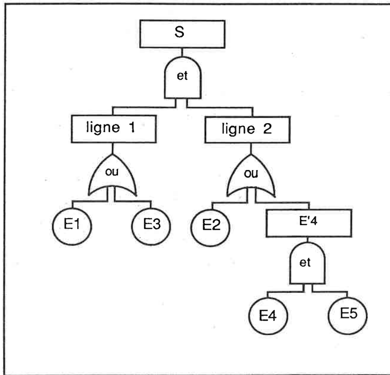
un exemple d'Arbre de Défaillance à partir du Diagramme de Fiabilité précédent
