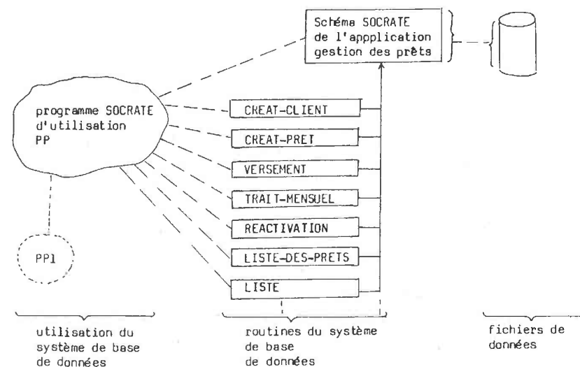
Structuration du système de base de données.
