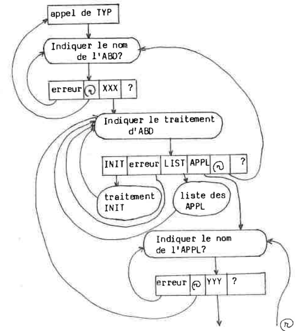
Schéma de l'automate d'états des commandes.
